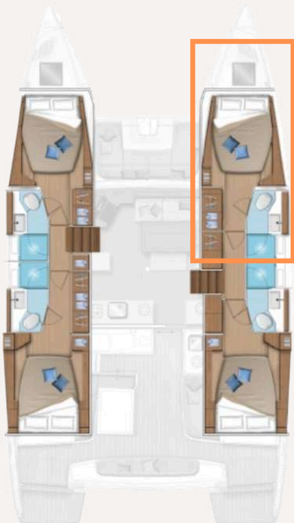
CABINES ÉQUIPAGE
